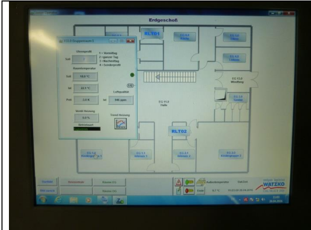
GLT-Darstellung Raumregelung
