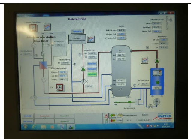
GLT-Anlagenbild Heizung
