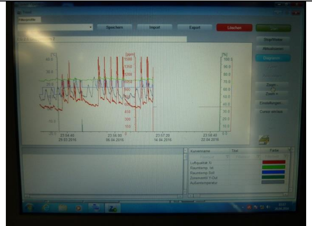
GLT-Trend-Darstellung
